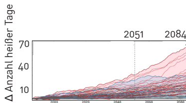
Prognose der Zunahme an heißen Tagen (über 25°C) in Darmstadt, (Climate Service Center Germany 2021)
